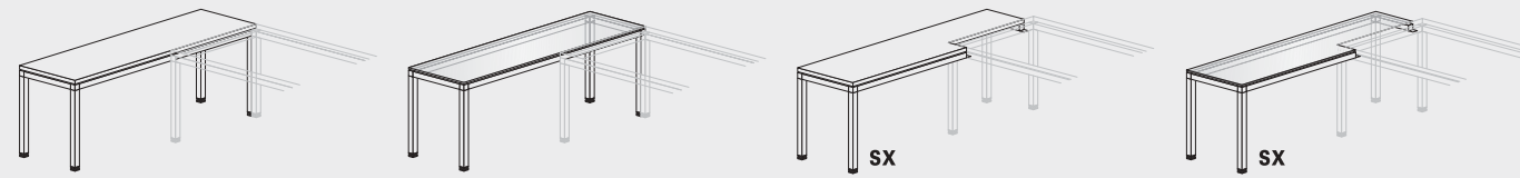
TL0419 L200 P60,8 H73÷75 TC0419 L200 P60,8 H73÷75 TL0420V L200 P60,8 H71,4÷73,4 TC0419V L200 P60,8 H71,4÷73,4 TL0424 (Dx) L200 P60,8 H73÷75 TL0423 (Sx) L200 P60,8 H73÷75 TC0424 (Dx) L200 P60,8 H73÷75 TC0423 (Sx) L200 P60,8 H73÷75 TL0424V (Dx) L200 P60,8 H71,4÷73,4 TL0423V (Sx) L200 P60,8 H71,4÷73,4 TC0424V (Dx) L200 P60,8 H71,4÷73,4 TC0423V (Sx) L200 P60,8 H71,4÷73,4
