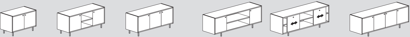
SDM 7202 cm. 104 x 47 x 67,2/73,2 h. SDM 7326 cm. 149,8 x 47 x 67,2/73,2 h. SDM 7302 cm. 149,8 x 47 x 67,2/73,2 h. SDM 7426 cm. 204 x 47 x 67,2/73,2 h. SDM 7408 cm. 204 x 47 x 67,2/73,2 h. SDM 7402 cm. 204 x 47 x 67,2/73,2 h.
