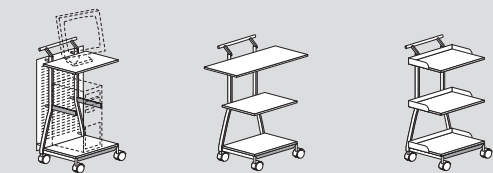
KC91548 cm. 46 x 55 x 92 h. KC91538 cm. 66 x 55 x 92 h. KC91508 cm. 46 x 55 x 92 h.
