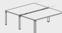
TV5514 L140 P164,7 H72 TV5516 L160 P164,7 H72 TV5518 L180 P164,7 H72 TV5520 L200 P164,7 H72
